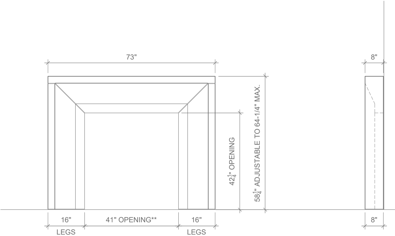
1 FRONT SCALE: 1/2"=1'-0"
